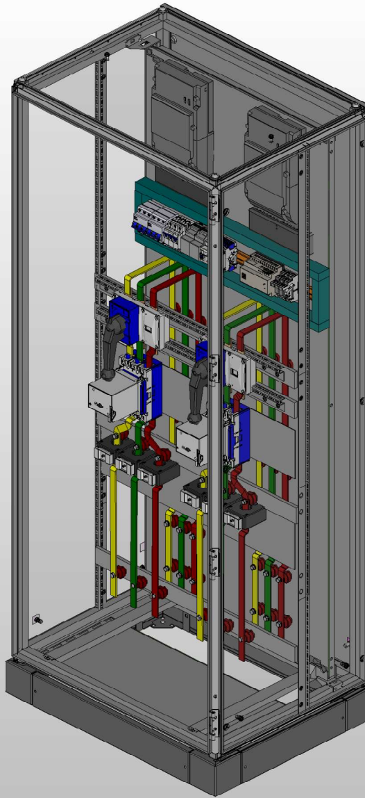
Вид без двери
